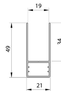
Pliszé keret és also csavaros vezető sín
